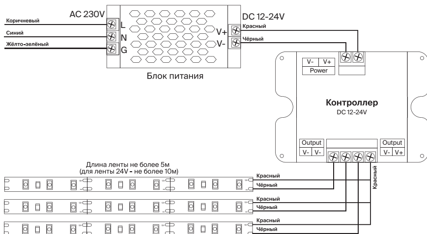
Рис. 1 схема подключения контроллера
