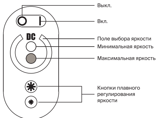
Рис. 2 назначение кнопок пульта управления
